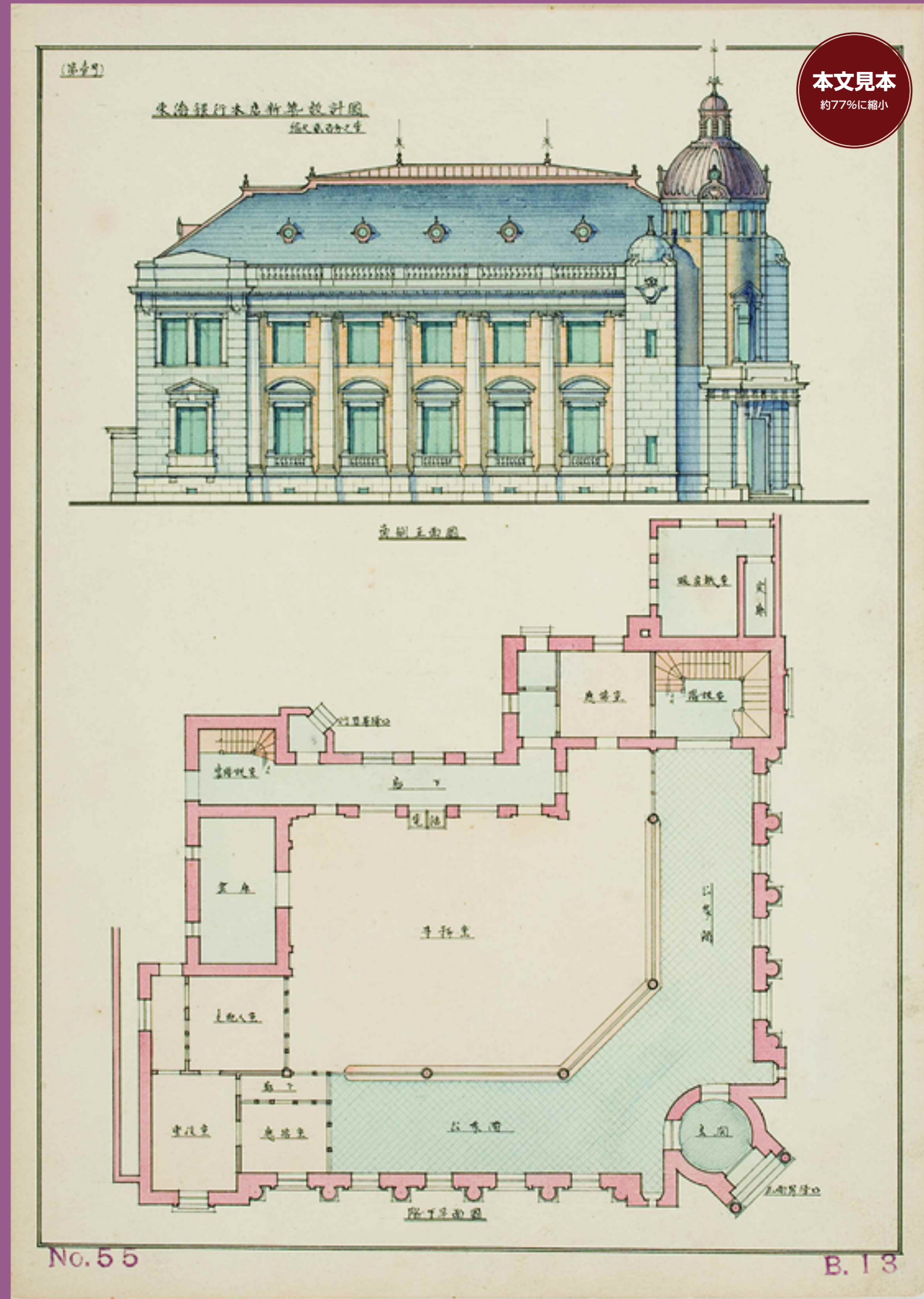
東海銀行本店新築設計図(第2巻所収)
