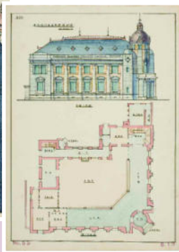
東海銀行本店新築設計図 (第2巻所収)
